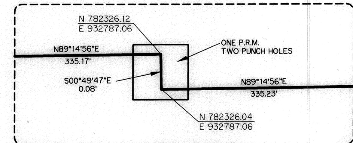
DETAIL "B" N.T.S.
