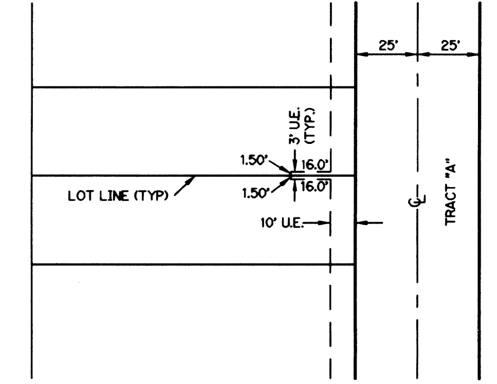
DETAIL "A" SCALE: 1"=40'
