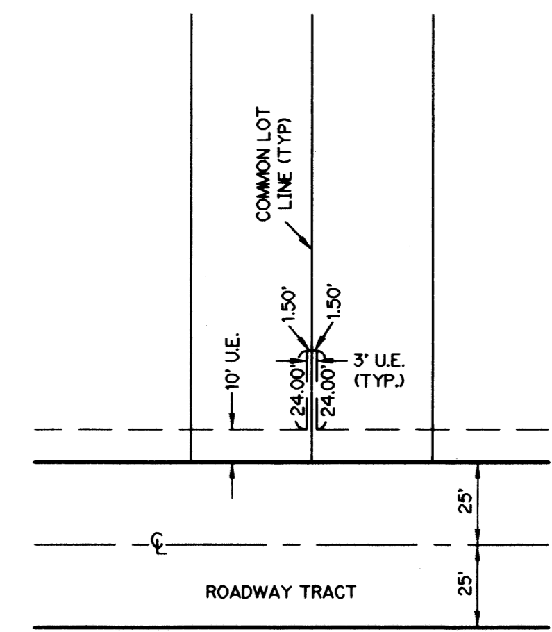
DETAIL "A" SCALE: 1"=40'
